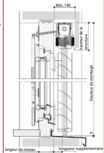
Montage de la structure
