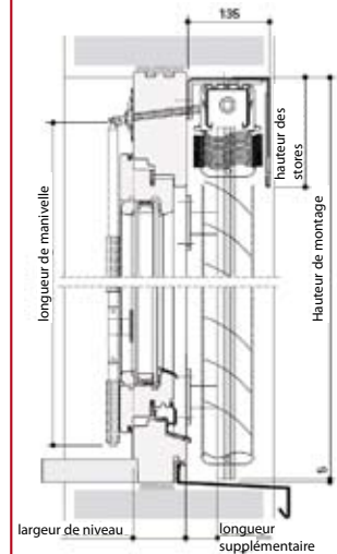
Montage des stores
